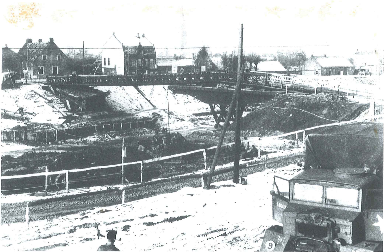
Baileybrug over Brug Vijftien, begin 1945. Let op de lage waterstand van de Zuid-Willemsvaart. De sluisen waren op diverse plaatsen vernield.
